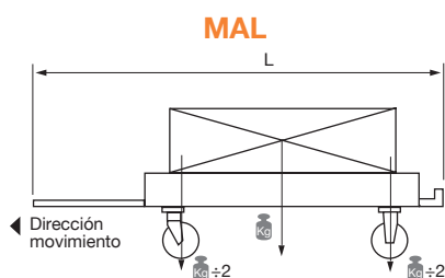
(1) Tracción mala, pero buena distribución de la carga entre rotantes delanteros y traseros.
