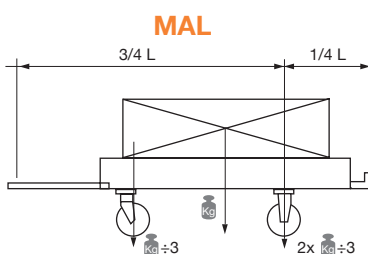
(2) Buena tracción, pero mala distribución de la carga entre rotantes delanteros y traseros.
