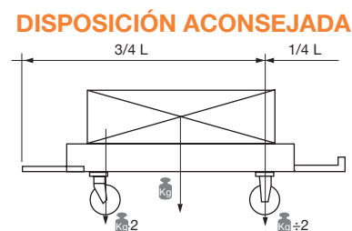
(2) Buena tracción y buena distribución de la carga entre rotantes delanteros y traseros.
